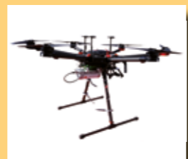
Drone Matrice 600 et Spectromètre MIRION
